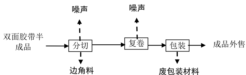
图 2-3 双面胶带生产工艺流程及产污位置图
